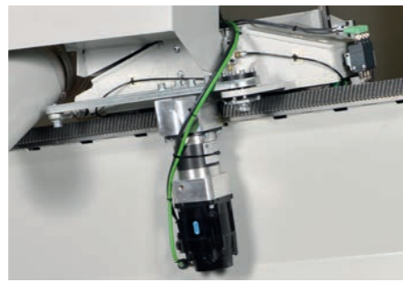
Top gantry motor
