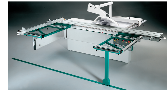
Option Carro squadratore doppio per pannelli pesanti / Double cross-cut carriage for heavy panels / Chariot équilibriseur double pour panneaux lourds / Doppel-Besäumschwenkarmrolltisch für schwere Platten / Carro ecuadorador doble para paneles pesados / Второй форматный стол для тяжелых панелей
